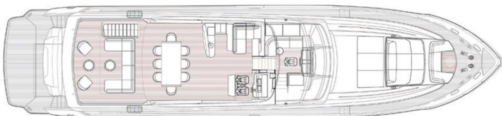
Flybridge
